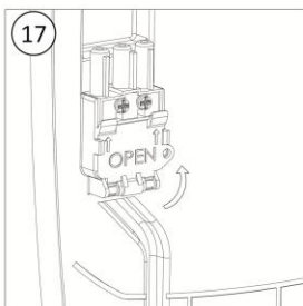
17 Cerrar la tapa de seguridad
