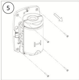
5 Desatornillar los tornillos de la pared (x4)
