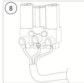
8 En la parte trasera del aparato, conectar los cables a la regleta siguiendo las letras marcadas en la regleta (N, L y Tierra)
